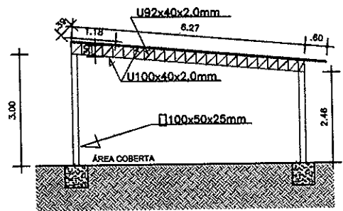
02 ELEVACÃO/CORTE S/ESCALA
